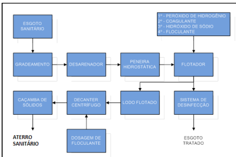
Figura 2-1: Fluxograma do Sistema de Tratamento
