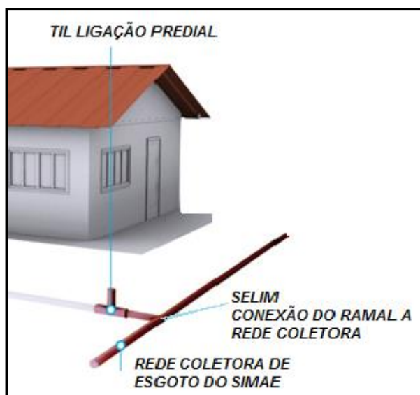
Figura 4-1: Representação da Ligação de um Ramal predial
