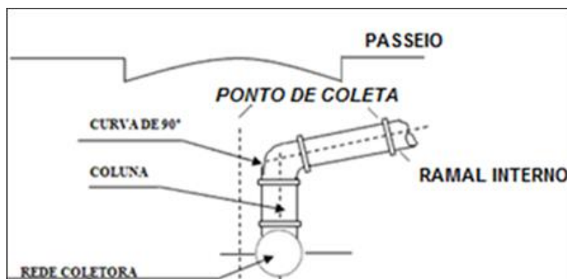
Figura 6-2- Representação da Ligação do Ramal predial
