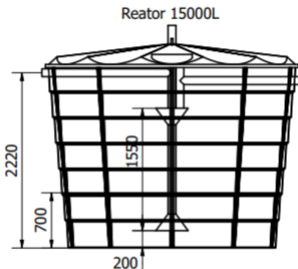
Figura 01 - Exemplo do Biorreator em PRFV.
