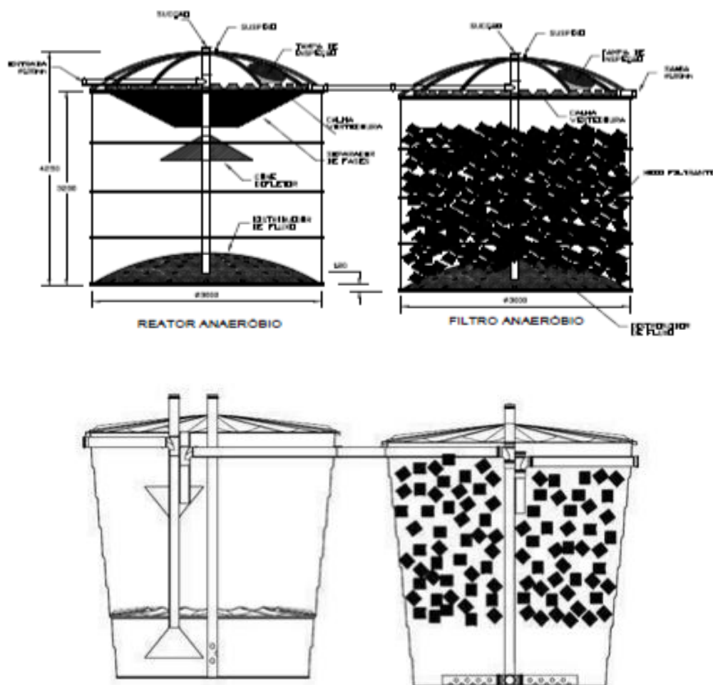
Figura 03 - Sistema Biorreator e Biofiltro em PRFV.
