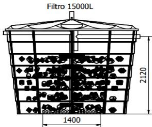
Figura 02 Biofiltro de 15000L em PRFV.
